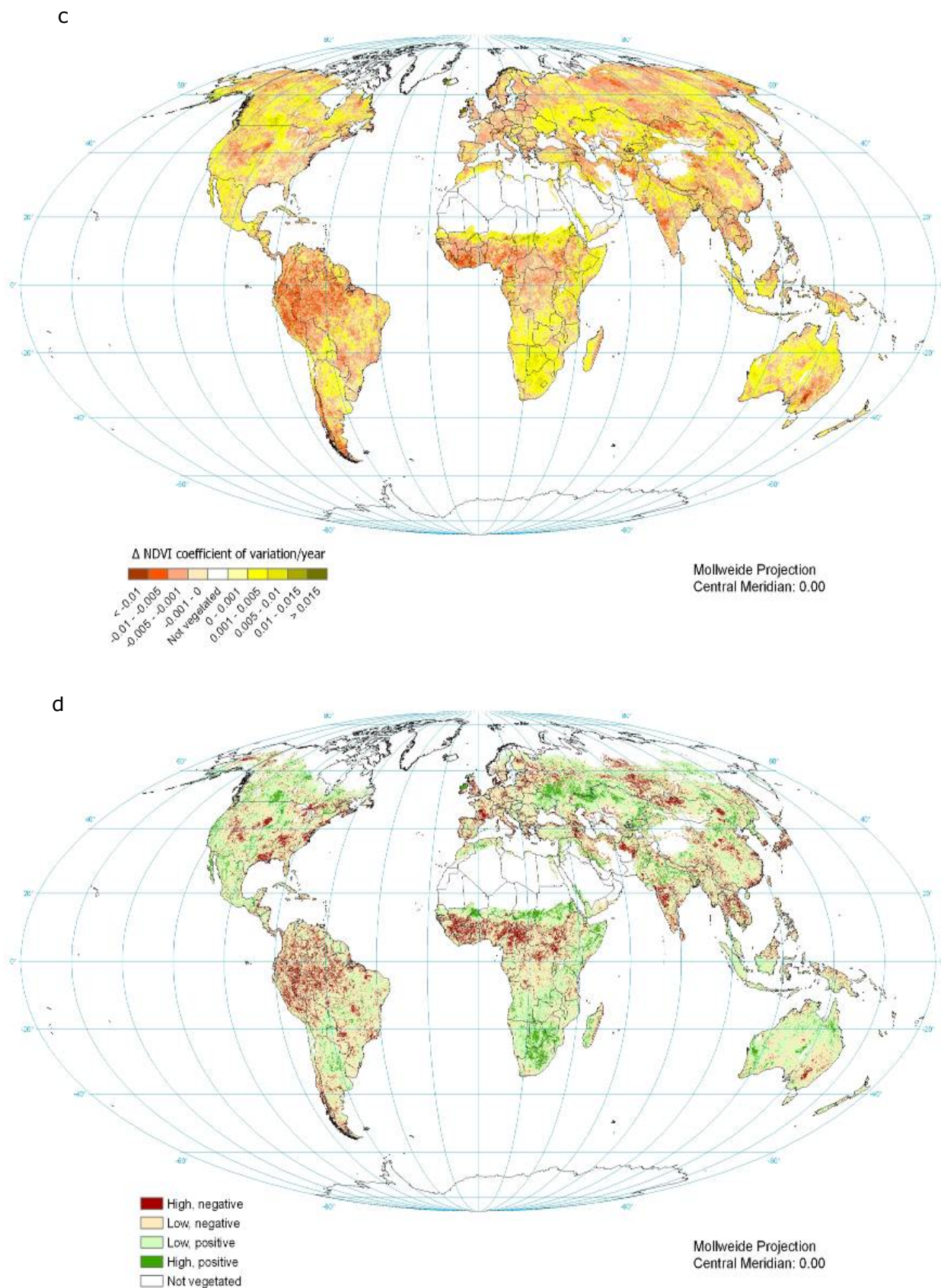
Figure S7. NDVI coefficient of variation 1981-2003: Trends (c – absolute) and confidence (d)
