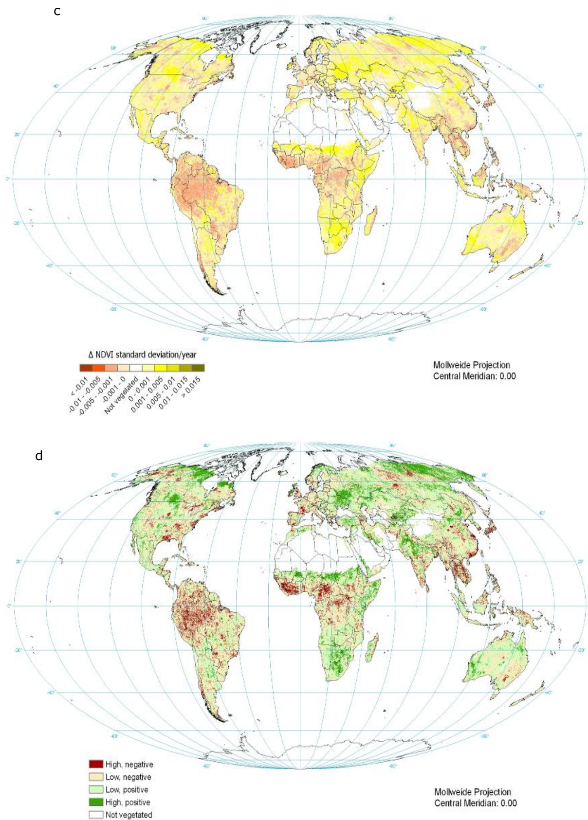
Figure S6. NDVI standard deviation 1981-2003: Trends (c – absolute) and confidence levels (d)
